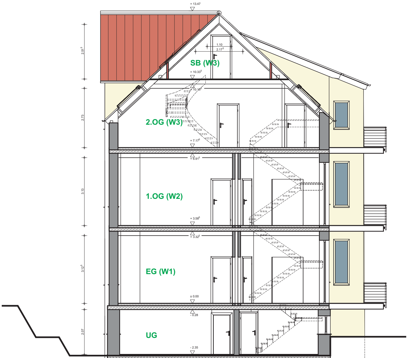
Schnitt 1:100
