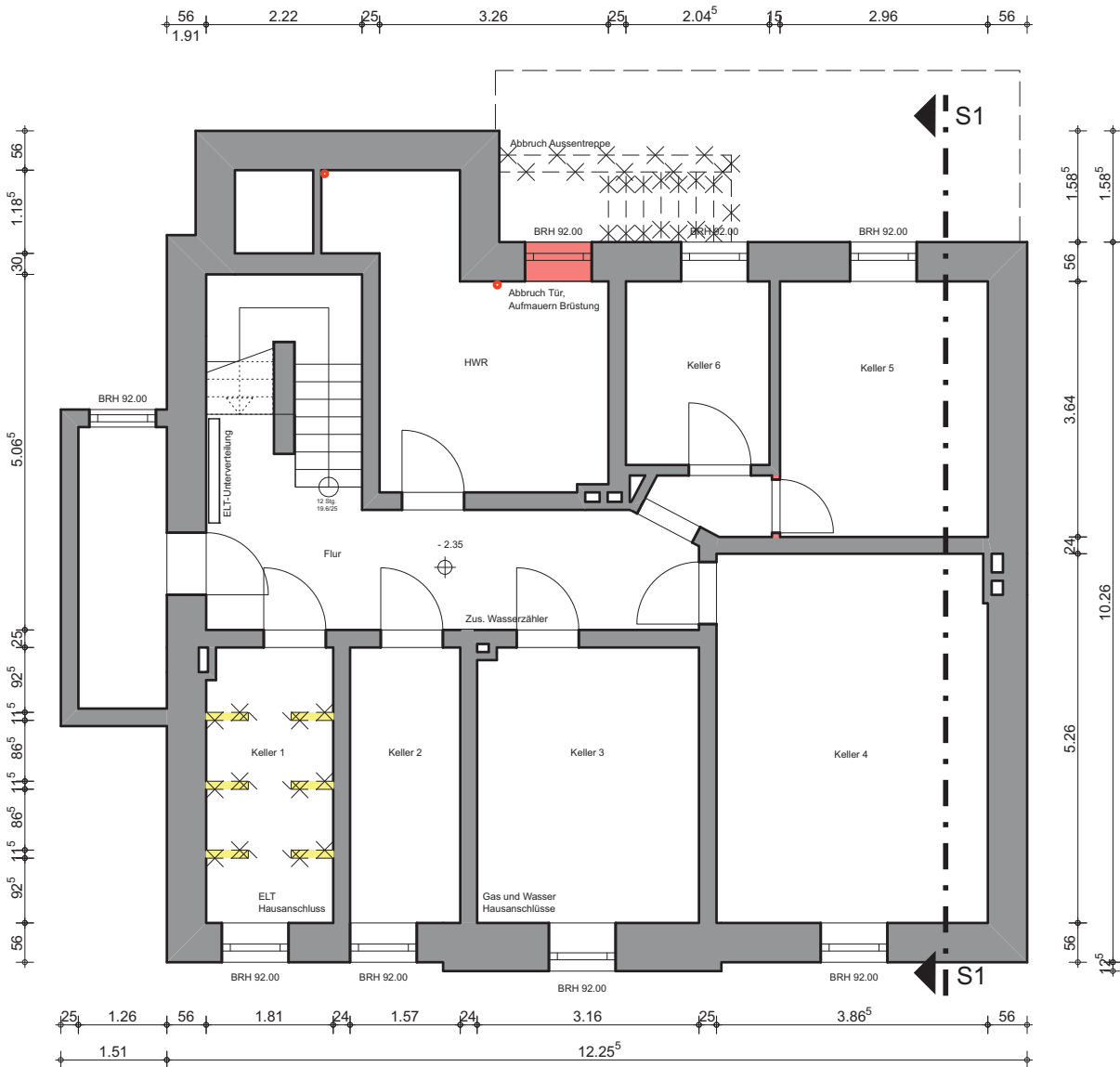
Grundriss UG 1:100
