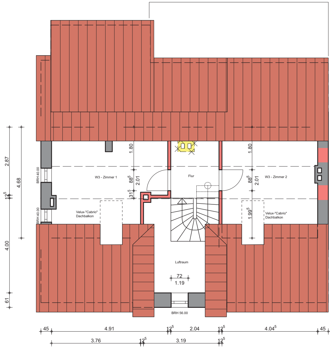
Grundriss DG 1:100
