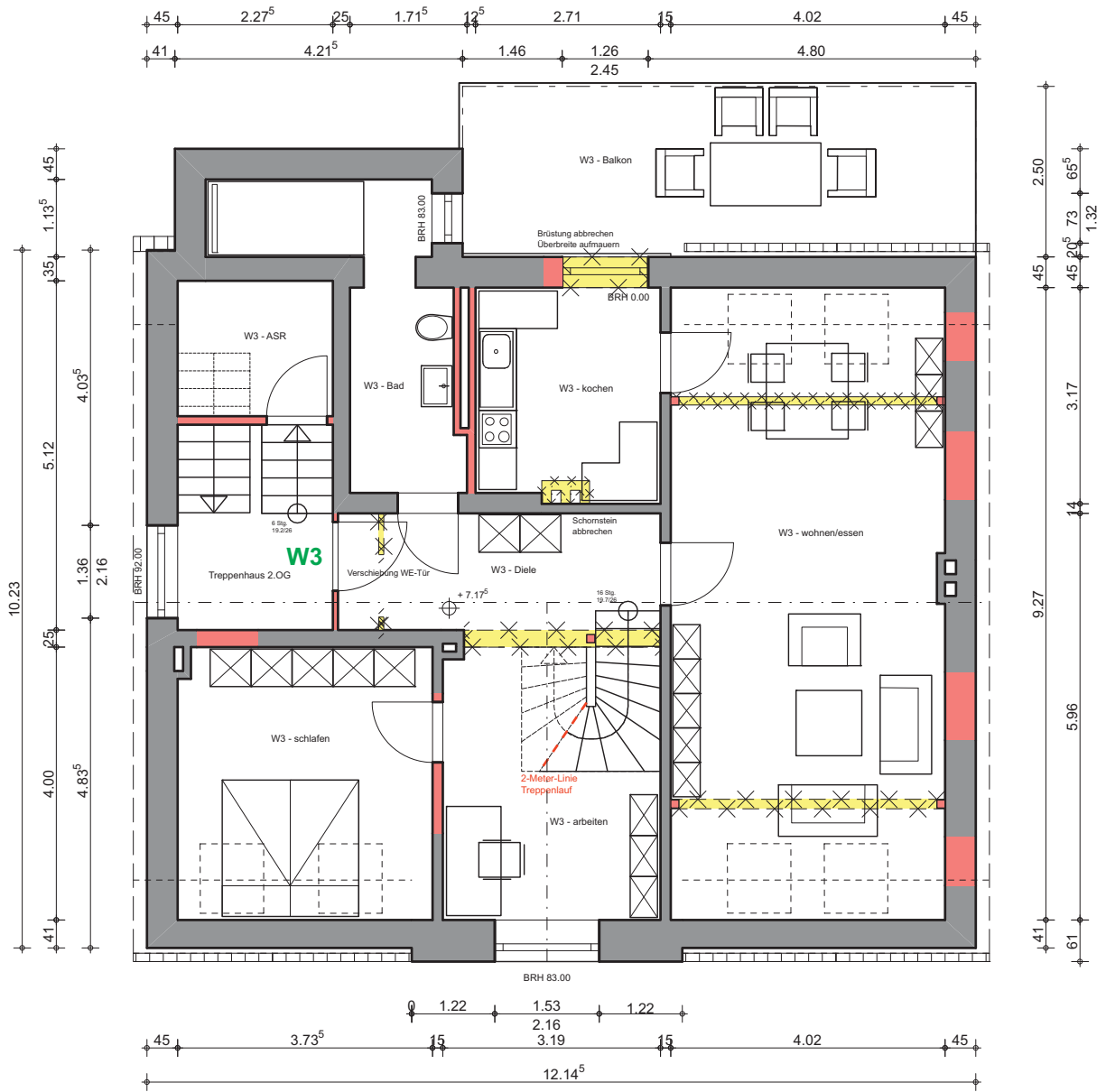
Grundriss 2.OG 1:100
